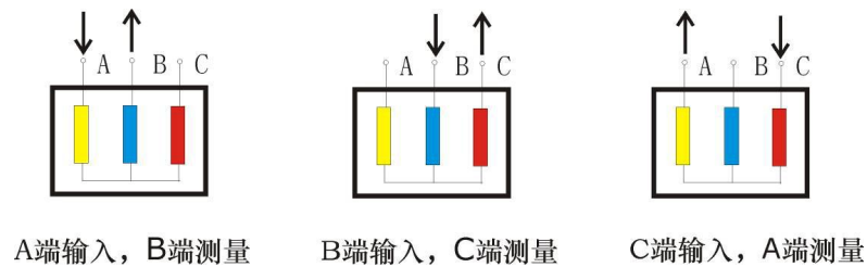
图 4 Y 接线
