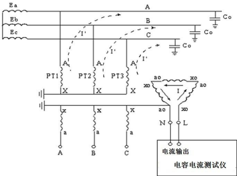
图 1 测量原理图
